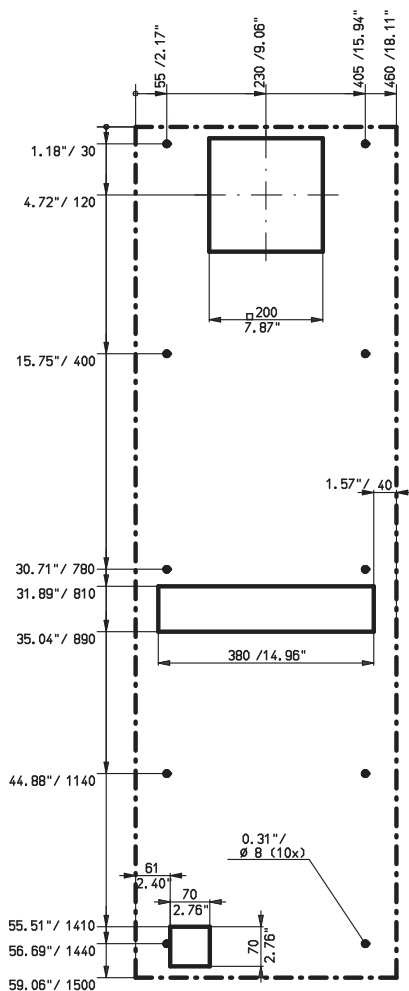
Lochbild: Schrank-Anbau
